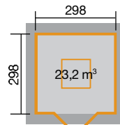
Gr. 2 mit Dachaufsatz 177.3030.10.00
