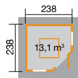
Gr. 1 mit Dachaufsatz 149.2424.10.00
