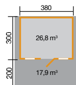
Vordach 200 cm inkl. Stützen, Abschluss- blende und Querstrebe
